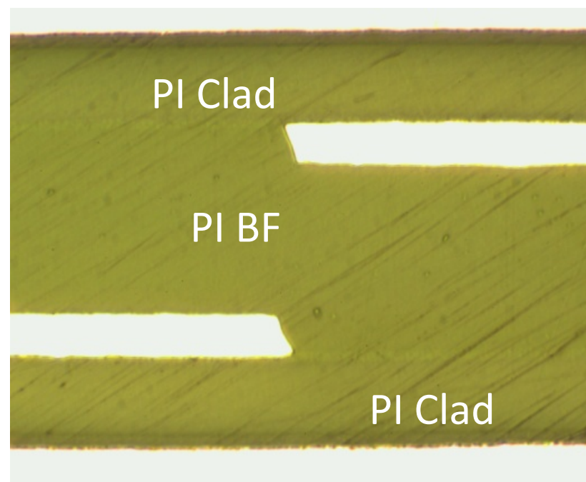
Bondply
