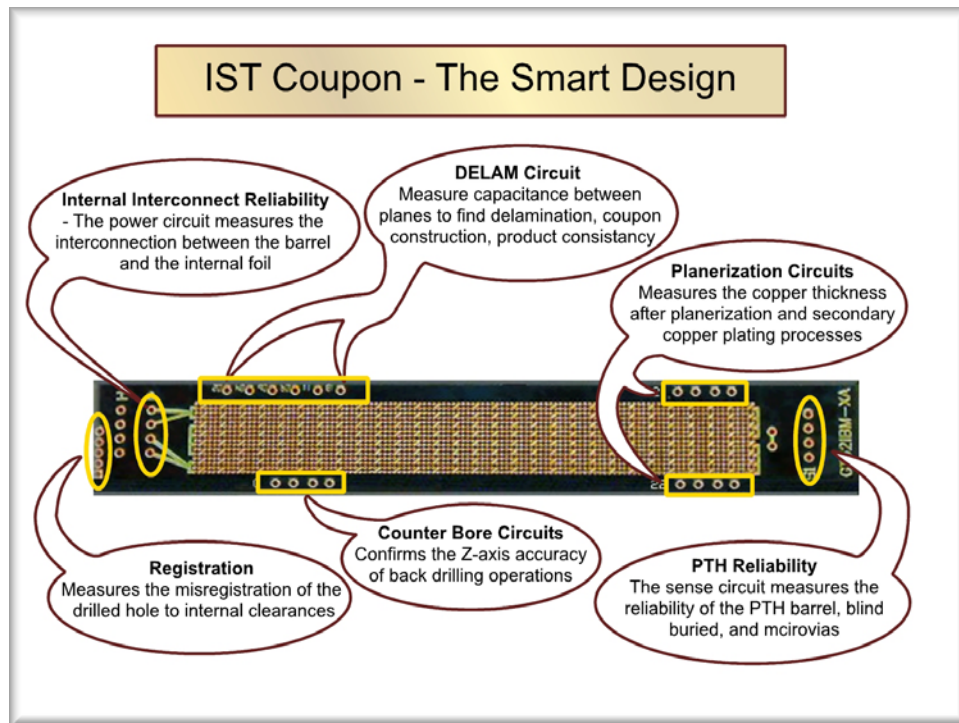
Figure 3 – IST Coupon
