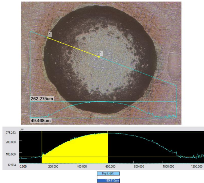
c. Solder Height = 189.410 um
