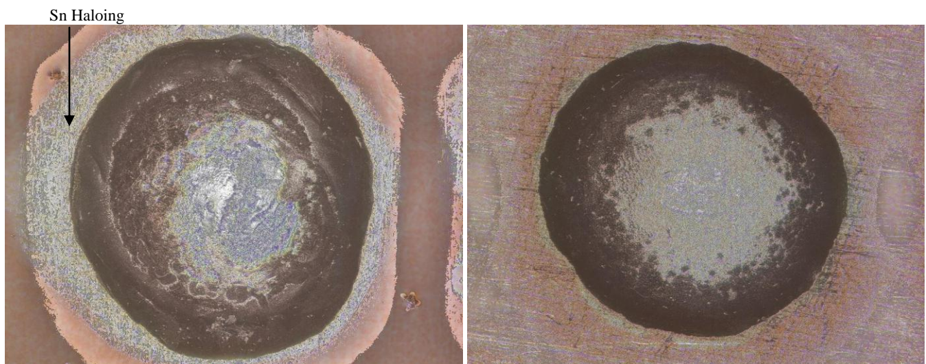
a. Vapor Phase Reflow
