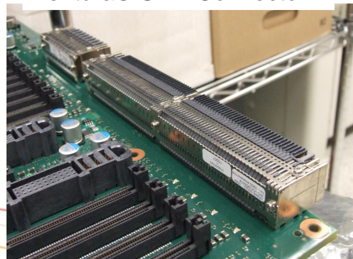
Ventura© SMT Connector
