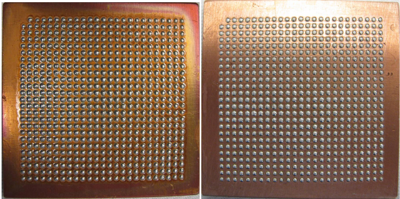
a. Vapor Phase Reflow
