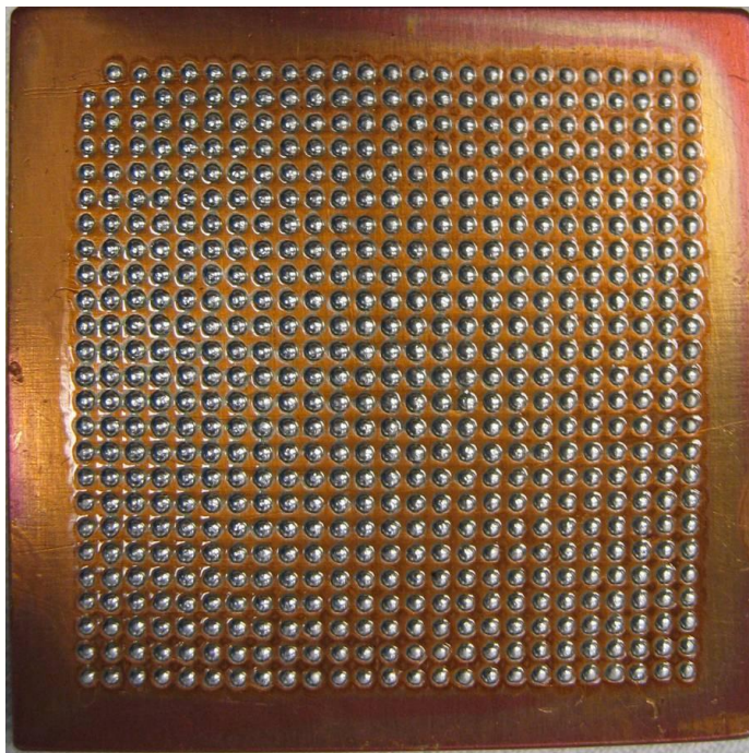
Vapor Phase
