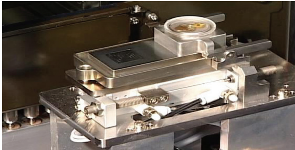
Linear Fluxer
